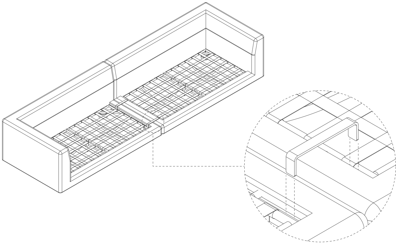
F. Connector 2pcs /SKU
